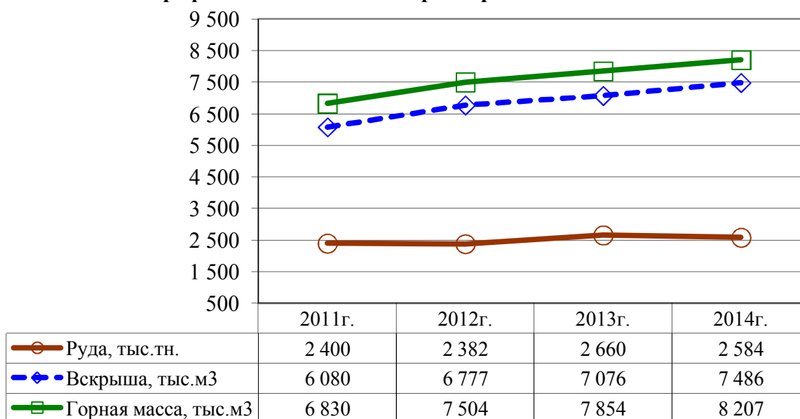
График №1 Выполнение горных работ по годам
