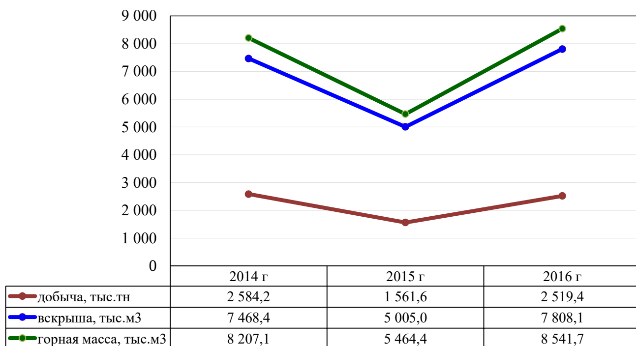
График №1 Выполнение горных работ по годам
